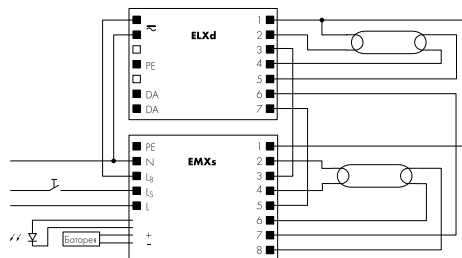
работа с 2 лампами – диммирование с ЭПРА ELXd
