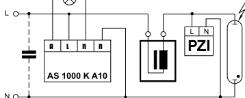
Пусковой переключатель для HI ламп, напряжением зажигания 0,9 кВ
