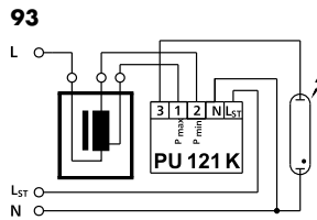
93 Фаза управления включена (L ST = 230 В) ПРА с двумя отводами
