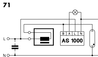
71 Пусковой переключатель для НМ ламп с вспомогательной лампой
