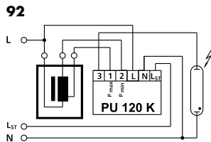
92 Фаза управления отключена (L ST = 0 В) ПРА с двумя отводами
