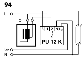
94 Фаза управления отключена (L ST = 0 В) ПРА с двумя отводами
