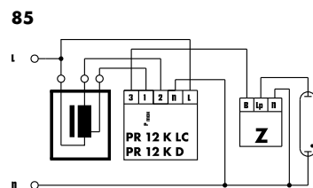
Электронное снижение мощности без фазы управления
