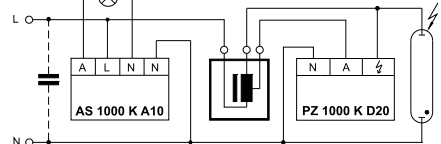
Пусковой переключатель для HS и HI ламп
