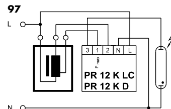
97 Электронное снижение мощности без фазы управления
