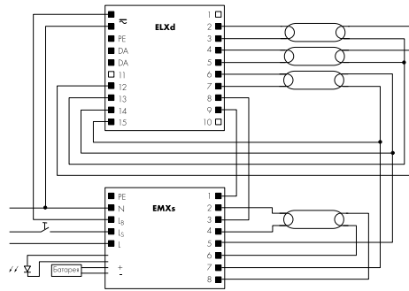
работа с 4 лампами – диммирование с ЭПРА ELXd
