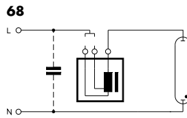
68 НМ лампы (ПРА с двумя альтернативными отводами напряжения)
