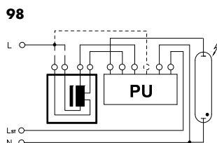
98 ПРА с двумя отводами мощности и двумя отводами напряжения (L ST = 0 В или L ST > 0 В)
