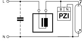
БЗУ для HI ламп, напряжением зажигания 0,9 кВ
