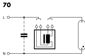
70 НМ лампы (ПРА с двумя альтернативными отводами мощности и напряжения)
