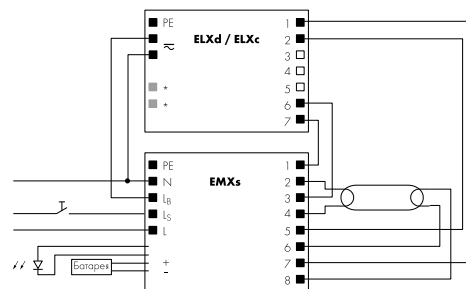
работа с 1 лампой – регулирование/ теплый старт с ЭПРА ELXd / ELXc
