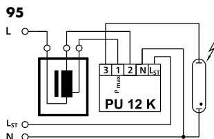
95 Фаза управления включена (L ST = 230 В) ПРА с двумя отводами
