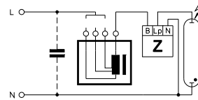
ИЗУ для HS и HI ламп (ПРА с тремя альтернативными отводами напряжения)
