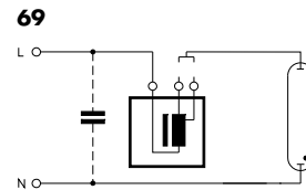
69 НМ лампы (ПРА с двумя альтернативными отводами напряжения)
