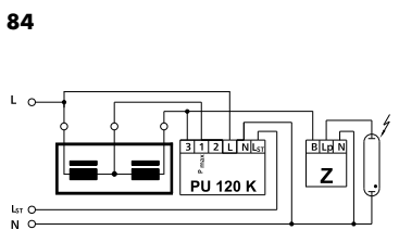
Фаза управления отключена (L ST = 0 В) с основной ПРА и дополнительной индуктивностью
