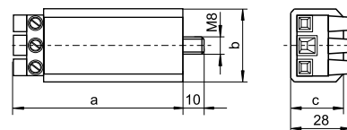
Корпус из поликарбоната – К
