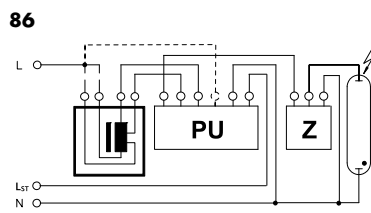
ПРА с двумя отводами мощности и двумя отводами напряжения (L ST = 0 В или L ST > 0 В)
