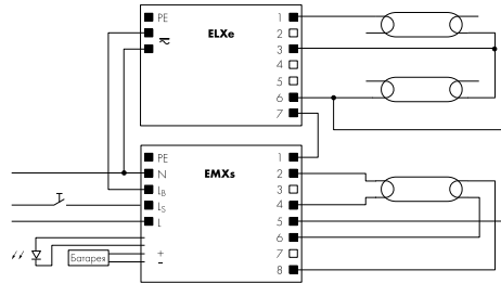
работа с 3 лампами – холодный запуск с ЭПРА ELXe
