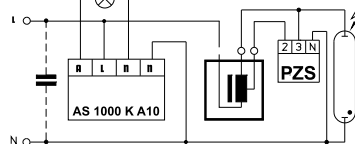
Пусковой переключатель для серийных HS ламп
