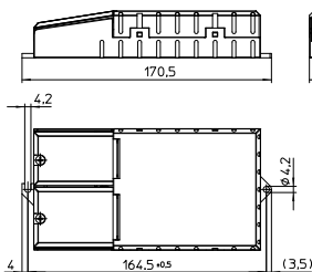
К34 с фиксатором кабеля
